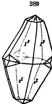
Calcite.
